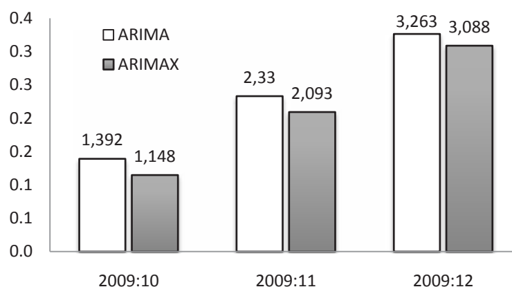
Rys. 12. Błędy ex ante prognoz liczby zarejestrowanych bezrobotnych dla modeli ARIMA i ARIMAX
